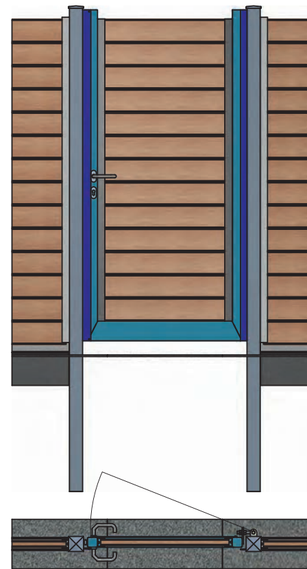
Låge set oppefra
